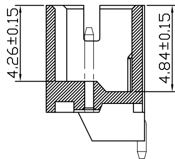
剖視圖 A-A
