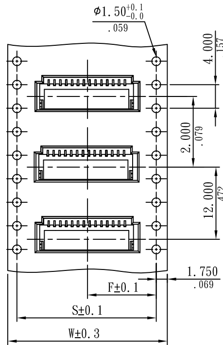
14~16(20) Circuits
